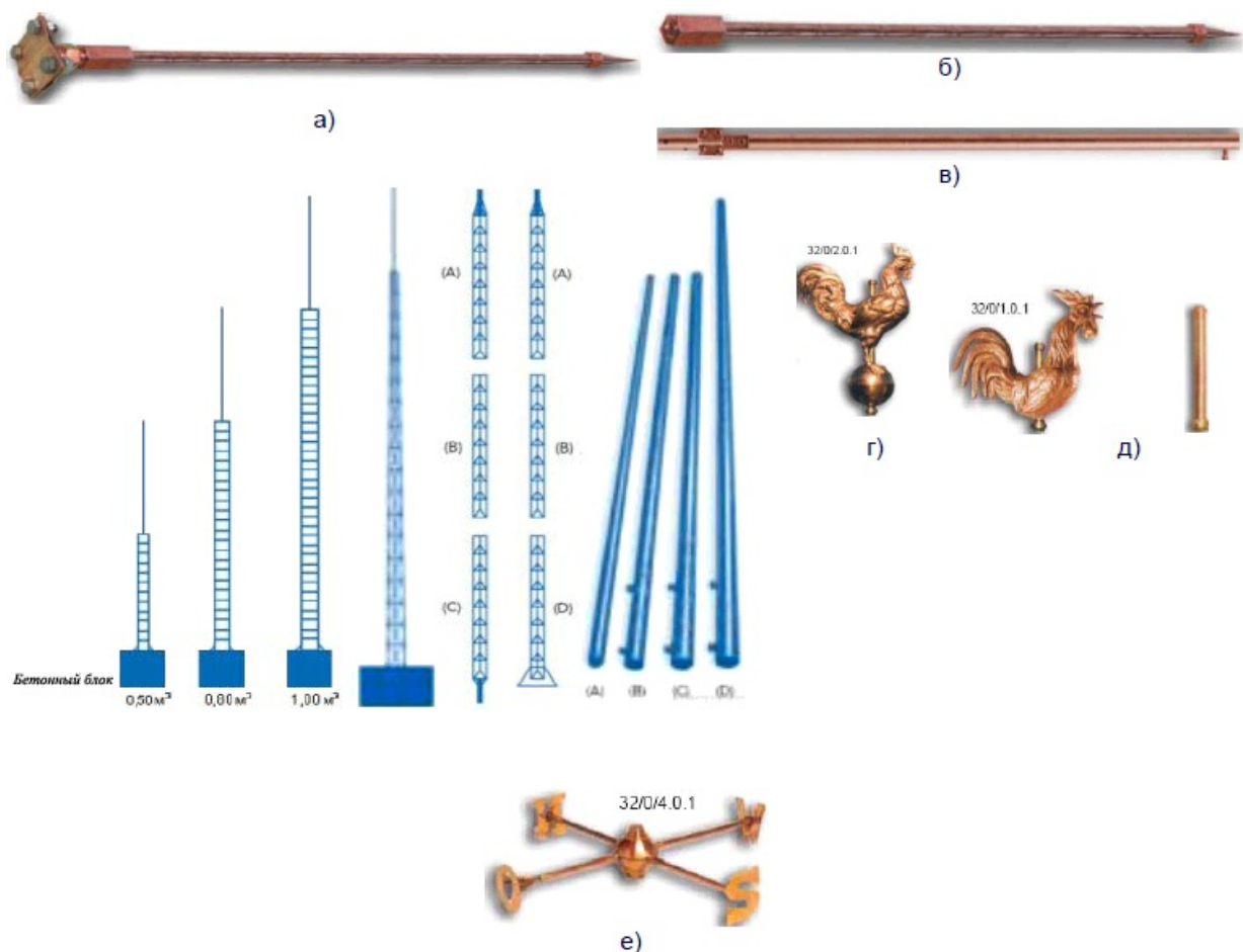
а), б), в) - заземлители; г), д), е) - декоративные элементы на молниеприемнике; ж) - легкие башенные опоры несущей конструкции; и) - башенная опора с проволочными оттяжками; к) - секции сборной легкой мачты несущей конструкции; л) - секции стойки телескопической.
