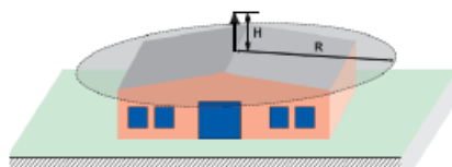
Рисунок 5 - Зона молниезащиты активного молниеприемника
