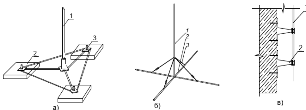
Рисунок 20 - Соединение активных молниеприемников при \Delta h \leq 1,5 м
