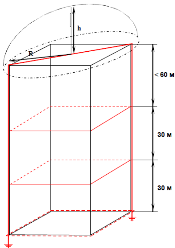
Рисунок 13 - Молниезащита здания из железобетонных конструкций выше 60 м
