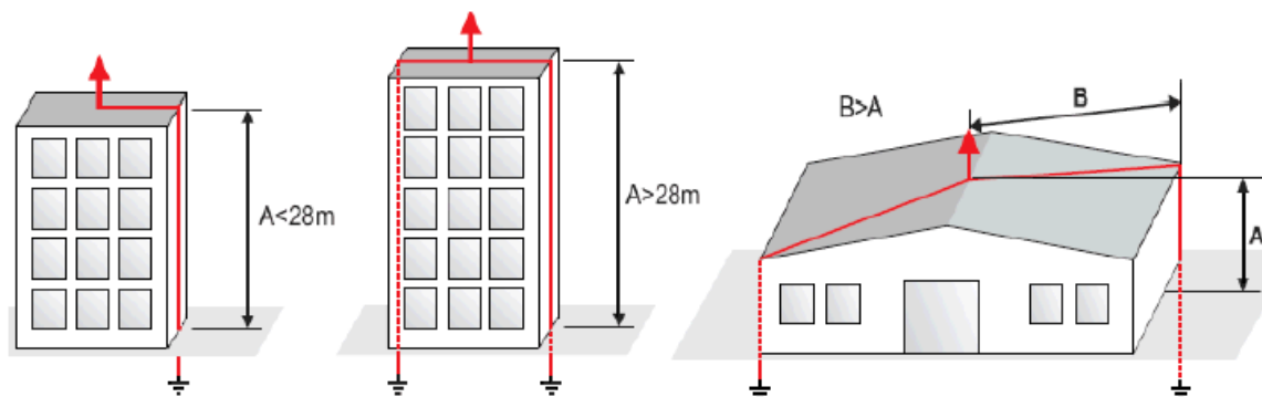
Рисунок 6 - Расчетная схема для выбора количества токоотводов
