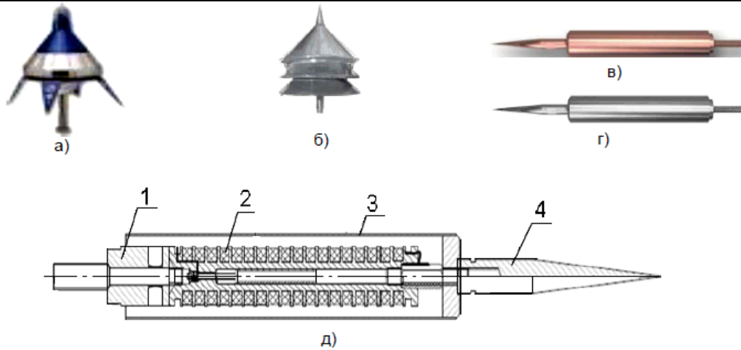
а) - Prevelectron 2 S6.60 ( \varnothing 185 мм, L = 385 мм); б) - Galactive 2 ( \varnothing 180 мм, L = 380 мм); в) - Громостар ( \varnothing 50 мм, L = 480 мм, медная); г) - Громостар ( \varnothing 50 мм, L = 480 мм, нержавеющая сталь); д) - устройство молниеприемной головки (Громостар); 1 - соединительное гнездо; 2 - блок сеток; 3 - корпус; 4 - острие.
