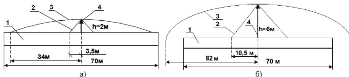
а) - классическая система молниезащиты; б) - система молниезащиты активного типа; 1 - объект; 2 - граница зоны защиты классической системы; 3 - граница зоны молниезащиты активного типа; 4 - молниеприемник на мачте;
