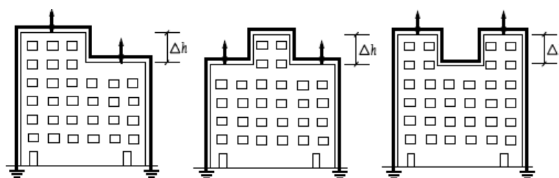
Рисунок 20 - Соединение активных молниеприемников при \Delta h \leq 1,5 м
