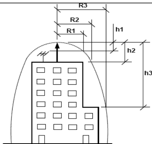
Рисунок 8 - Параметры охраняемой зоны
