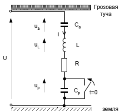
Рисунок 3 - Электрическая схема молниезащиты с упреждающей стримерной эмиссией
