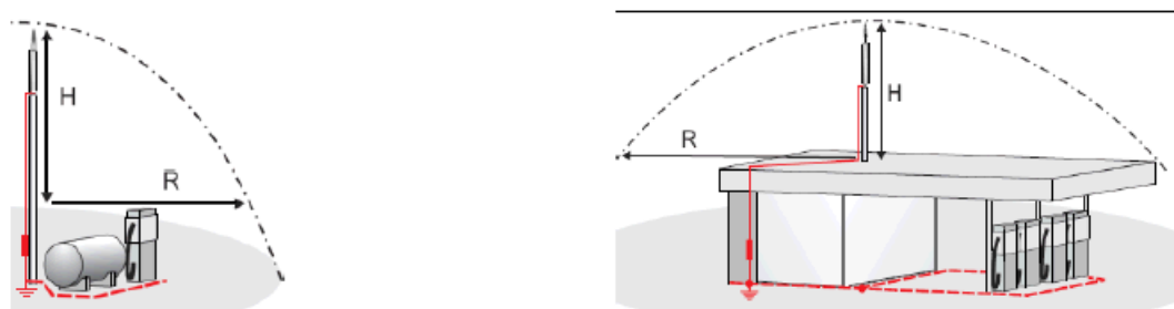
Рисунок 14 - Схема молниезащиты резервуаров с нефтепродуктами
