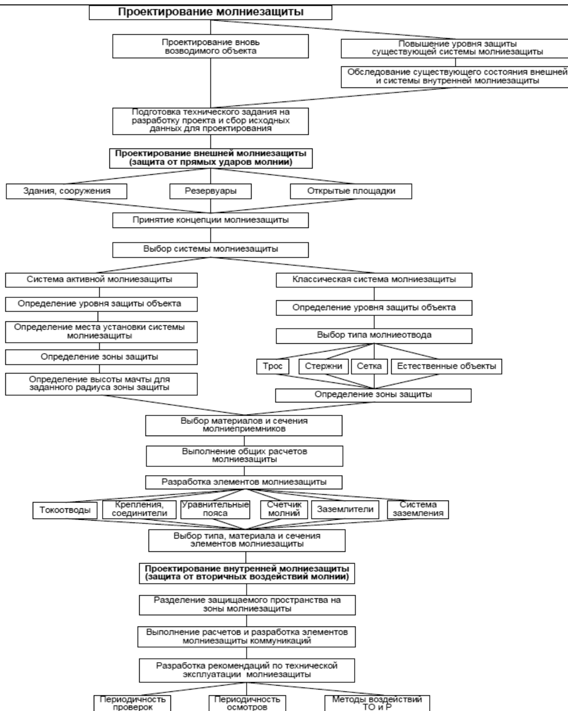
Рисунок 1 - Алгоритм процесса проектирования молниезащиты
