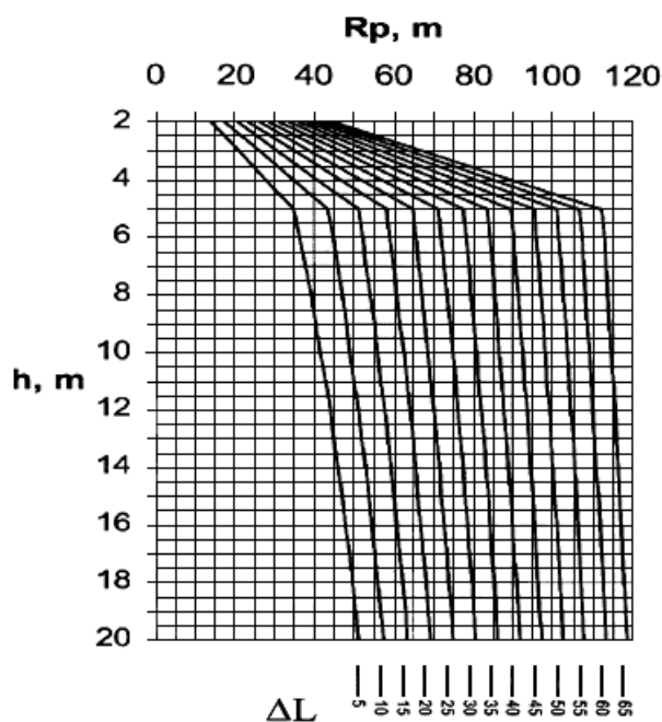
Диаграмма 2 - II категория защиты от молнии ( D = 45 м)
