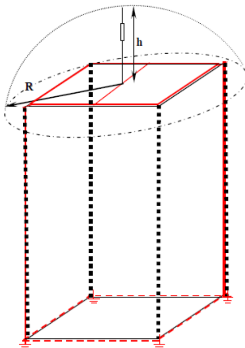
Рисунок 12 - Схема молниезащиты здания с металлическими элементами
