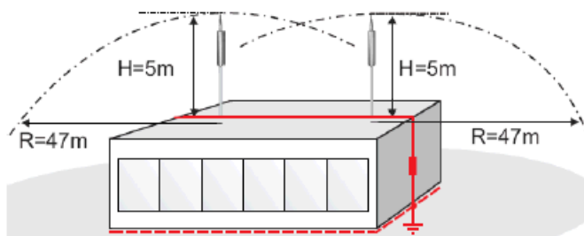
Рисунок 19 - Схема молниезащиты здания двумя молниеприемниками высотой установки 5 м
